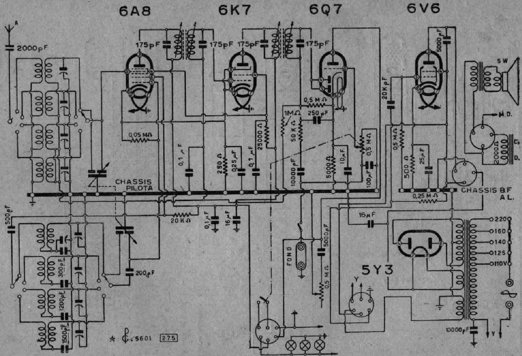
Lo schema elettrico del mod. 542
